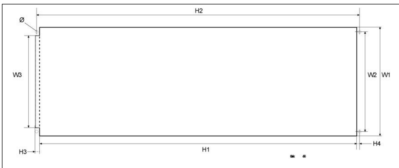
Figura 5-3. Orificiul necesar pentru montare cu flanșă, de la FR4 la FR6
