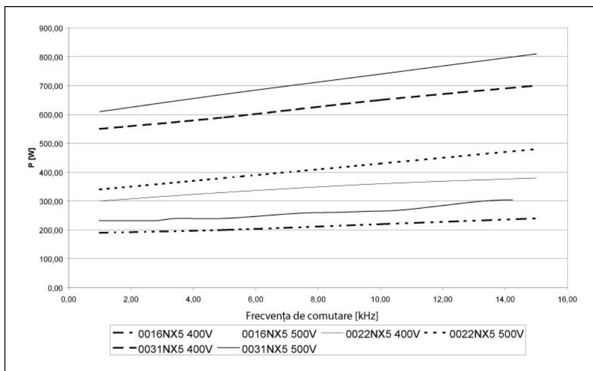
Figura 5-14. Pierdere de putere ca funcție a frecvenței de comutare; NX_5 0016...0031
