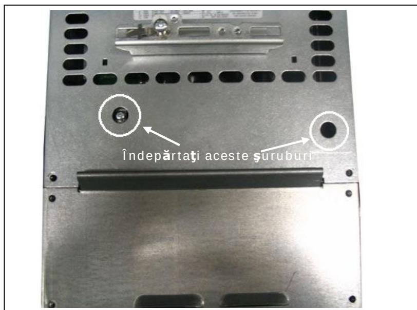
Figura 6-3. Modificarea clasei de protecție EMC, FR6. Nu este nevoie să îndepărtați capacul cablurilor
