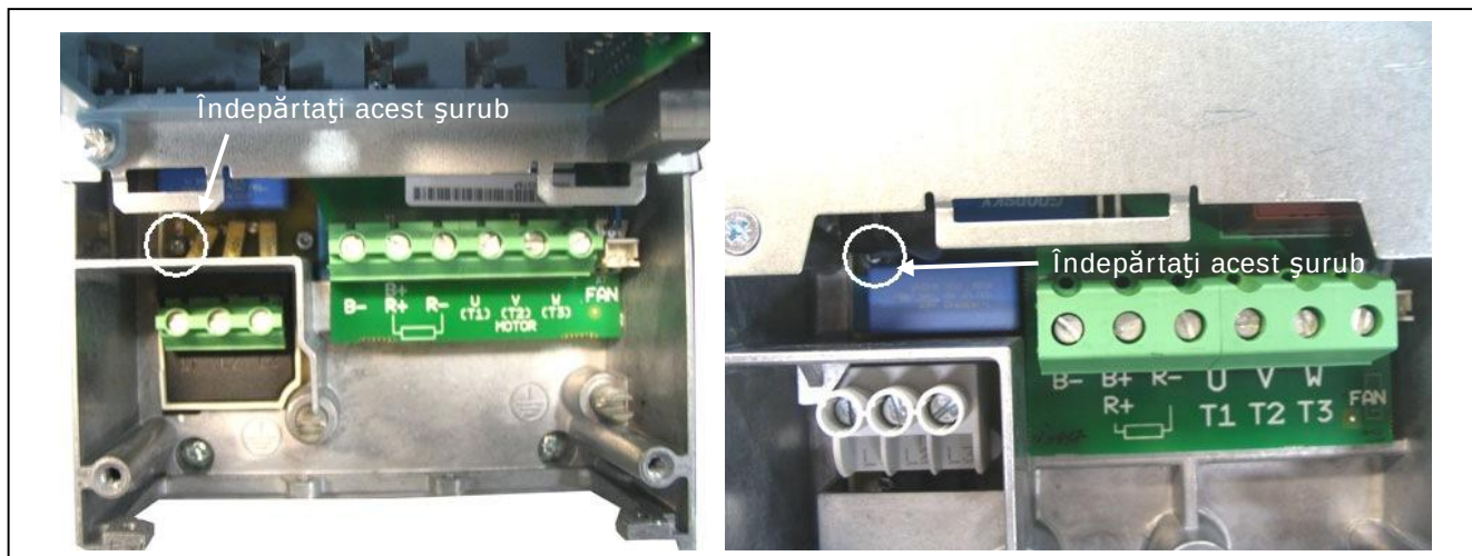
Figura 6-2. Modificarea clasei de protecție EMC, FR4 (stânga) și FR5 (dreapta). Mai întâi, îndepărtați capacul cablurilor
