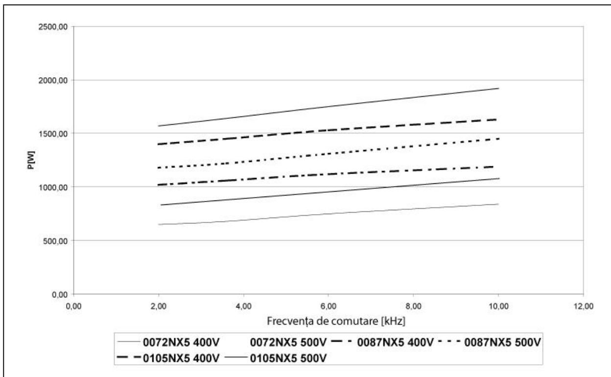
Figura 5-16. Pierderea de putere ca funcție a frecvenței de comutare; NX_5 0072...0105
