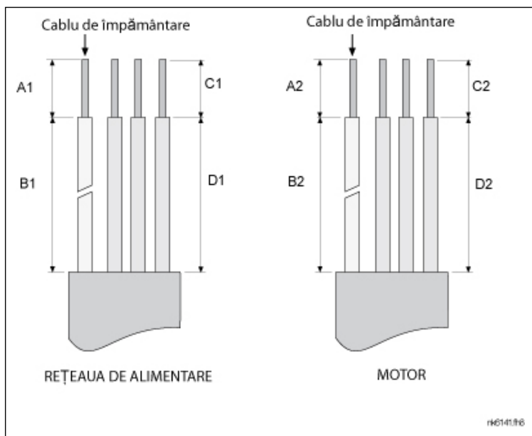
Figura 6-6. Dezizolarea cablurilor
