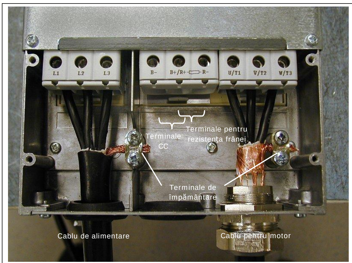
Figura 6-13 . Instalarea cablurilor la Vacon NXS/P, FR6
