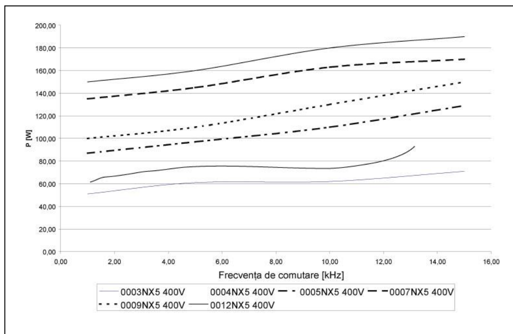
Figura 5-13. Pierdere de putere ca funcție a frecvenței de comutare; NX_5 0003...0012
