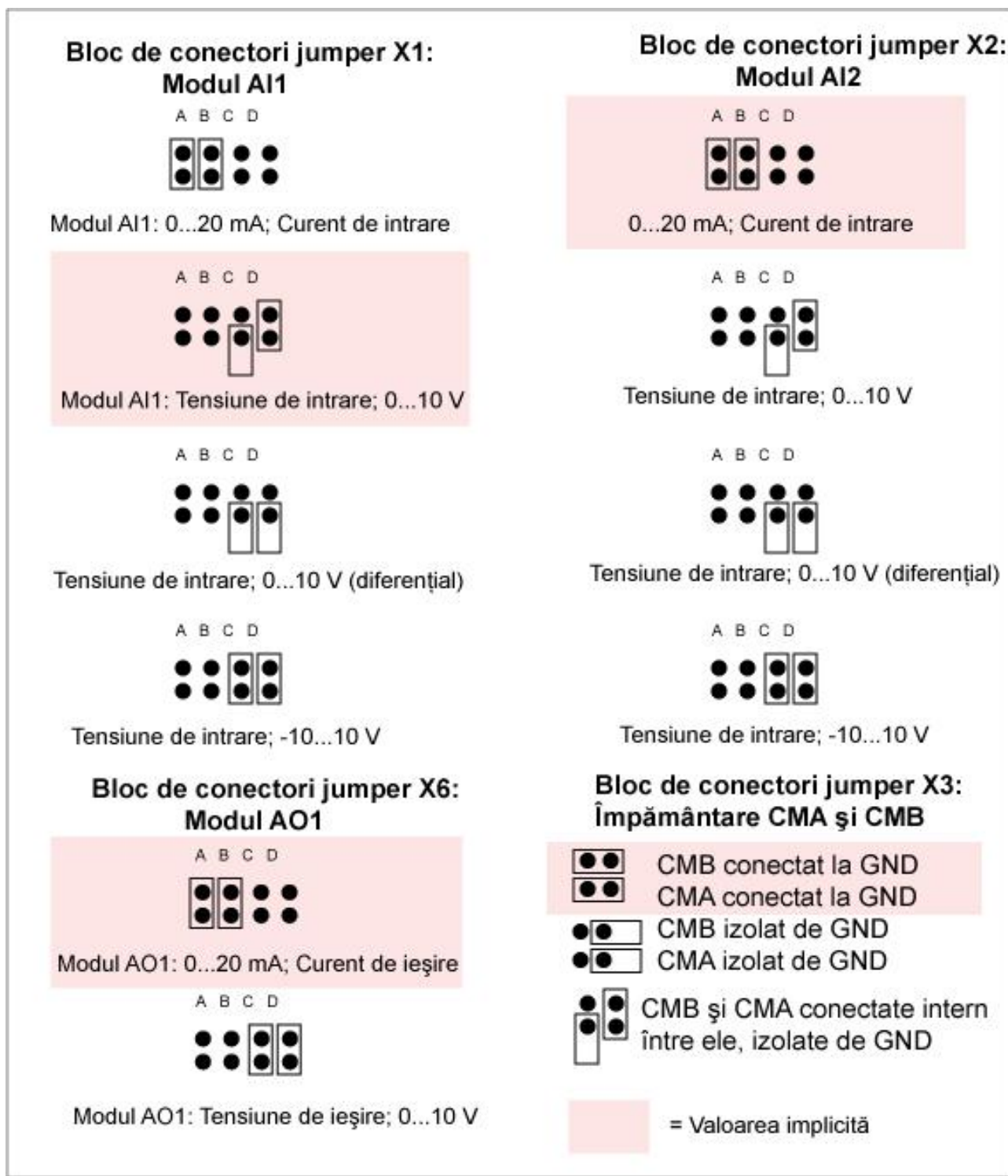
Figura 6-31. Selectare conectori jumper pentru placa OPT-A1
