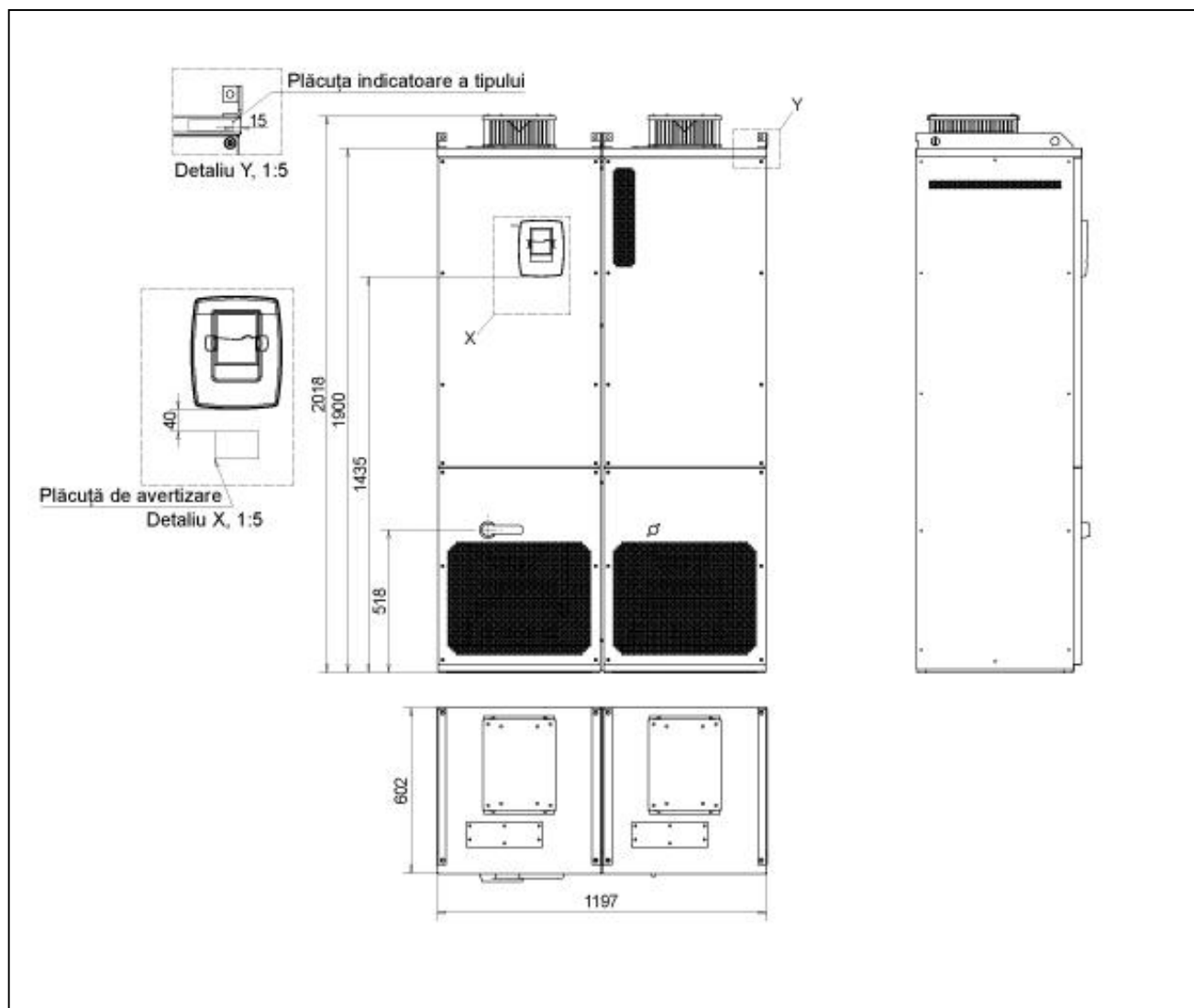
Figura 5-10. Dimensiuni Vacon NXP, FR12 (unități amplasate pe podea)
